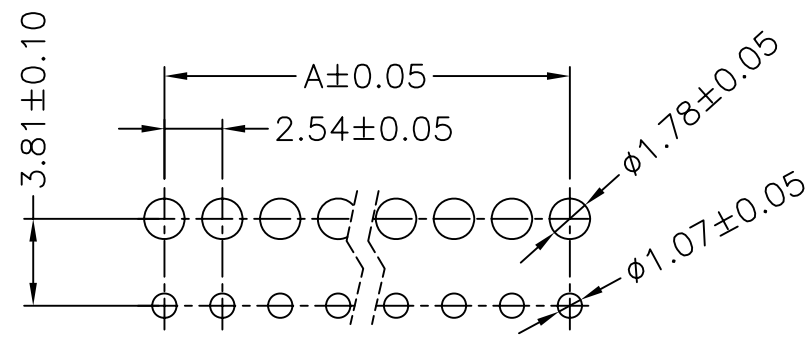
P.C.Board Layout
