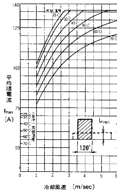
平均順電流—冷却風速 (方形波120°導通, 冷却体AH02-12)
