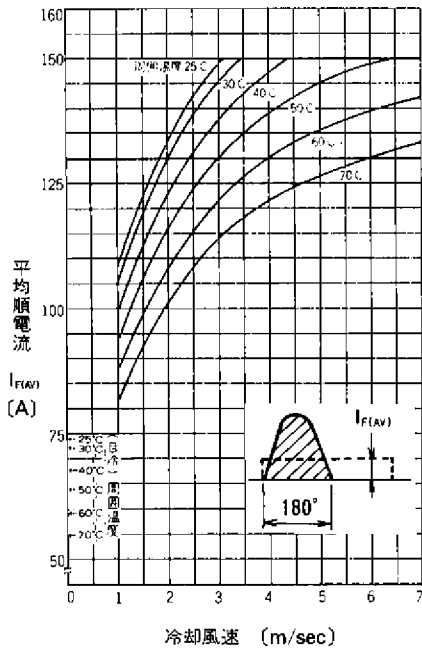
平均順電流—冷却風速 (正弦波180°導通, 冷却体AH02-12)
