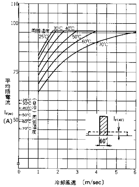
平均順電流—冷却風速 (方形波60°導通, 冷却体AH02-12)
