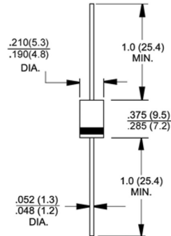
DO-201AD
