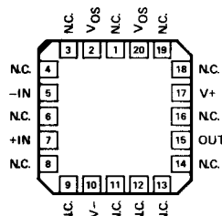
OP-77BRC/883 LCC (RC-Suffix)
