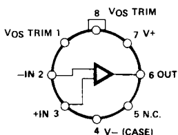
TO-99 (J-Suffix)
