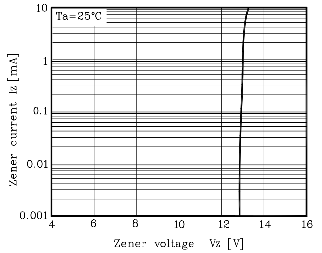
Fig. 2 I_Z - V_Z
