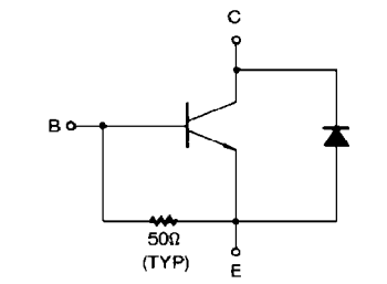
-EQUIVALENT CIRCUIT
