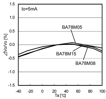
Fig.10 Ta - Vo
