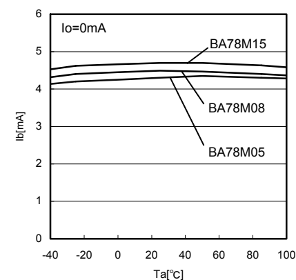
Fig.11 Ta - Ib
