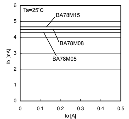
Fig.12 Io - Ib
