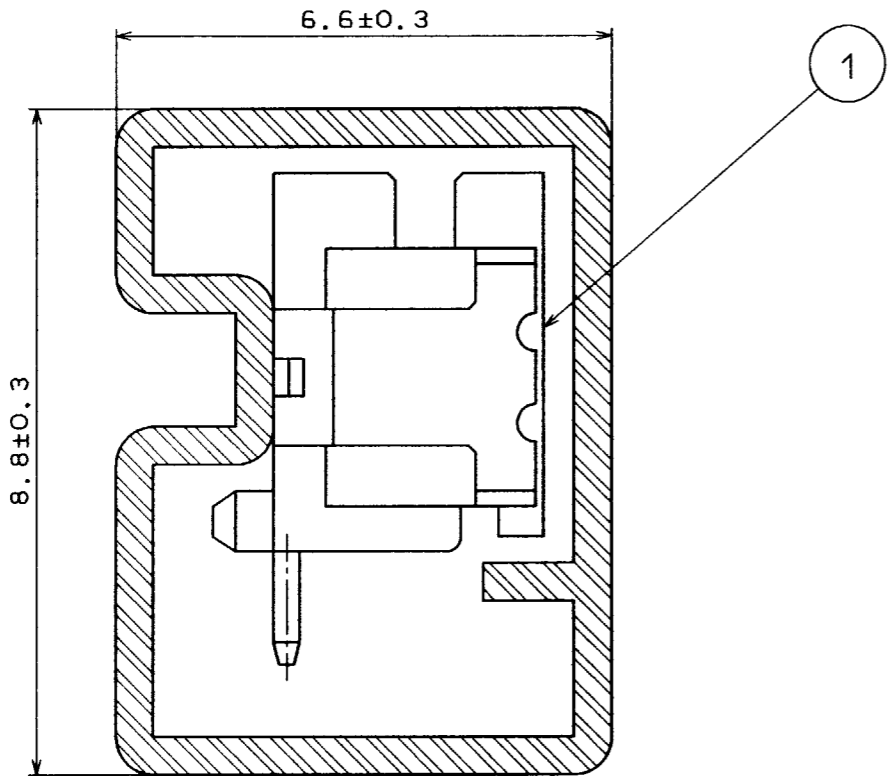
A-A (10:1)
