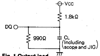
Fig. 1 Output load
