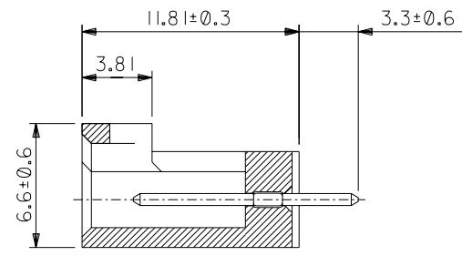
断面 X-X
