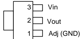
TO220-3L
