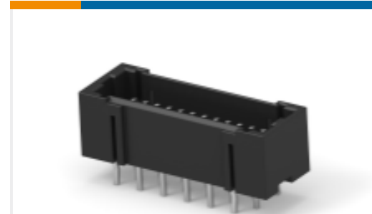
TE Part #4-292208-4 MINI CT D/R DIP 24P BLACK
