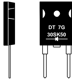
ACTUAL SIZE TO-247AC (TO-3PAC) PACKAGE
