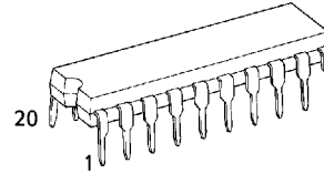
P (DIP20-P-300-2.54A) Weight : 1.30g (Typ.)
