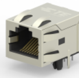
TE Part #3-2301994-8 RJ45 JACK INT.MAG. 10/100 1X1 INV.
