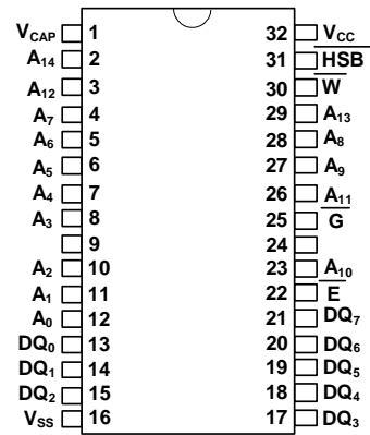
32 Pin SOIC
