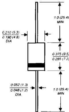
DO-201AD
