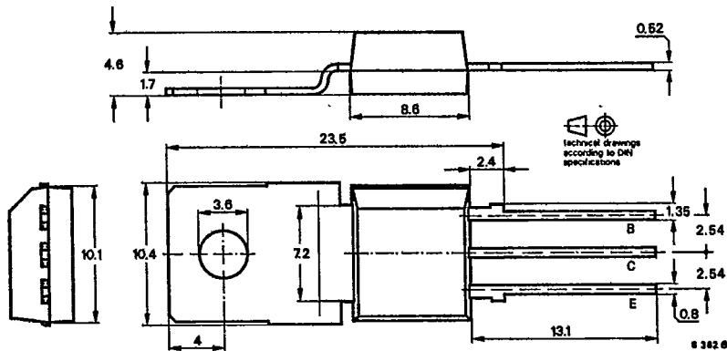
BF 870 SA · BF 872 SA
