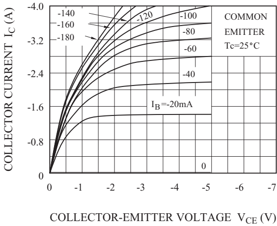
I_C - V_{CE}
