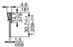
Plug-on cap, 1-pole Y 307 851 01
