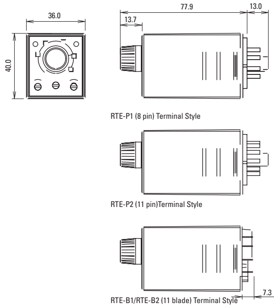
RTE-B1/RTE-B2 (11 blade) Terminal Style
