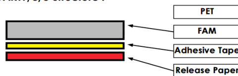
FAM1/3/5 Structure :
