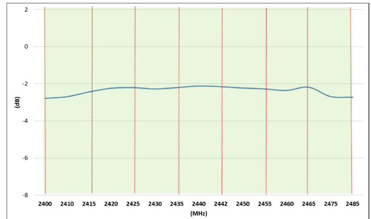
VSWR
