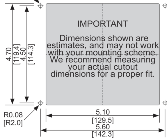
Cutout Dimensions
