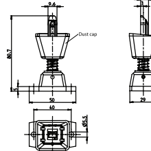
A3 ACTUATOR KEY 391.1702.230
