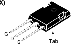
PLUS247 (IXFX)
