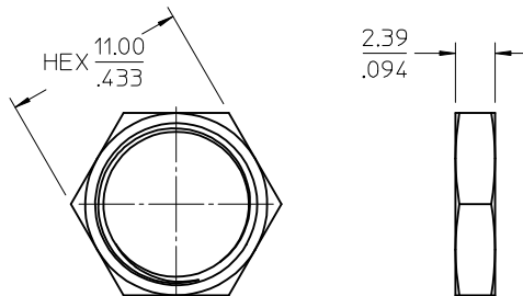
JAM NUT
