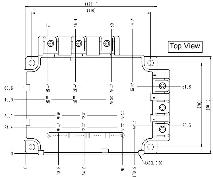
PM200RL1A060 350G
