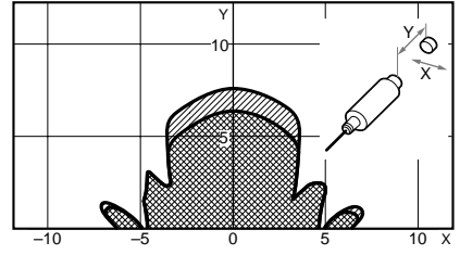
V600-D23P53 & V600-H52
