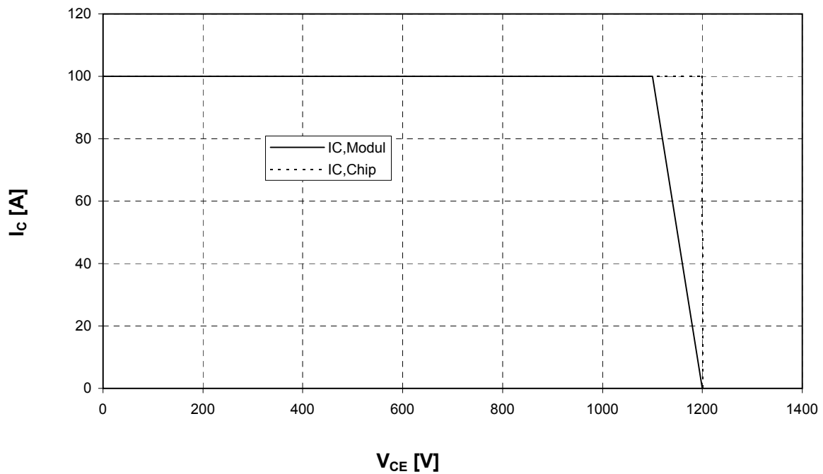
Sicherer Arbeitsbereich Wechsler. (RBSOA) I_c = f(V_{CE}) Reverse bias safe operating area Inverter (RBSOA) T_{vj} = 125^\circ\text{C} , V_{GE} = \pm 15\text{V} , R_G = 15 \text{ Ohm}
