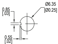
Keyway
