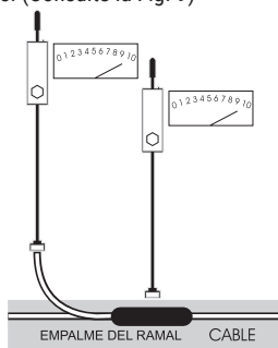
Fig. 7. Señal sobre el empalme de un ramal
