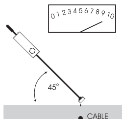
Fig. 2. Determinación de la profundidad
