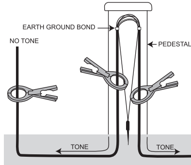
Fig. 10. Coupling Points
