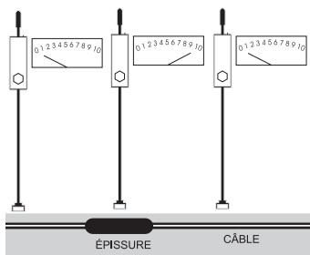
Fig. 6. Changements de signal au-dessus d'une épaisseur
