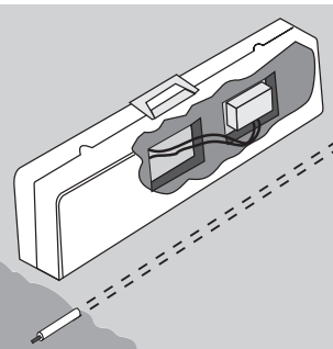
Fig. 15. Ubicación de la antena para distancias largas
