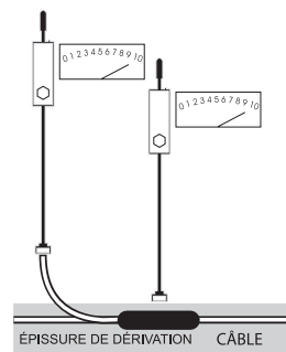
Fig. 7. Signal au-dessus d'une épaisseur de dérivation
