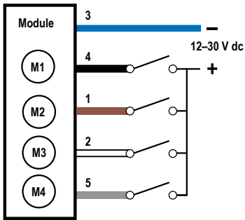
PNP Input
