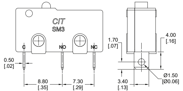
Solder Lug
