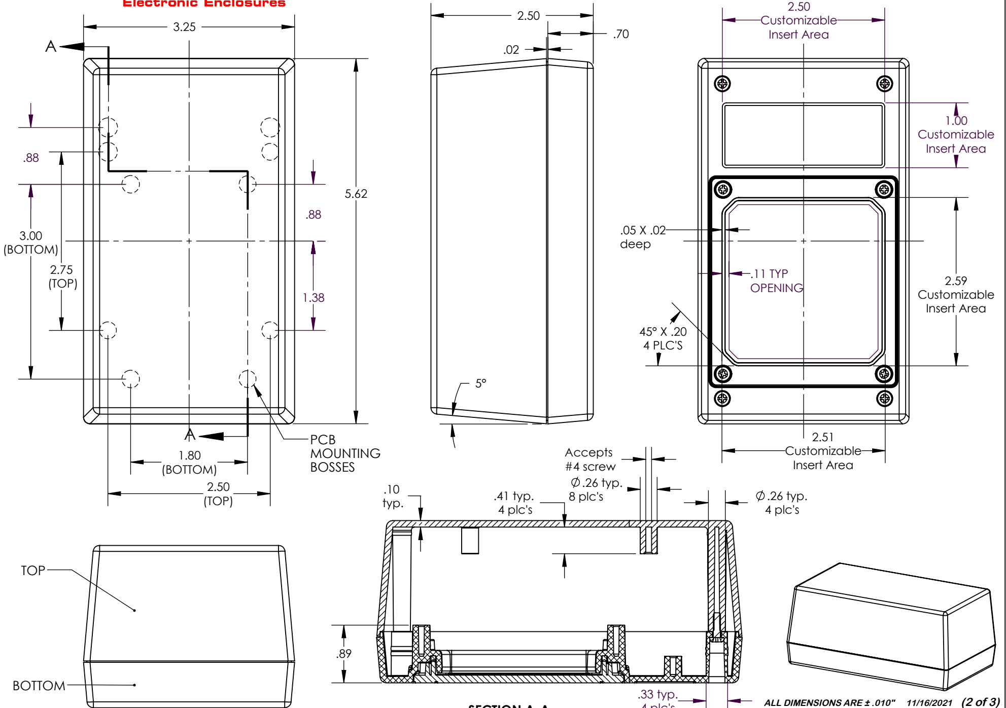
SECTION A-A
