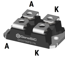
SOT-227
