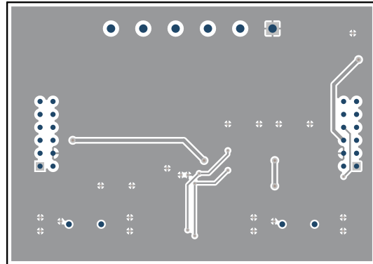
Figure 6-8. SENS063 Bottom Layer
