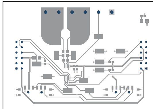
Figure 6-6. SENS063 Top Layer
