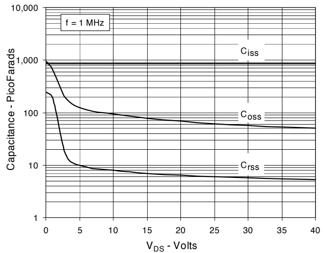
Fig. 10. Capacitance
