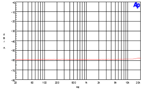
17. CMRR
