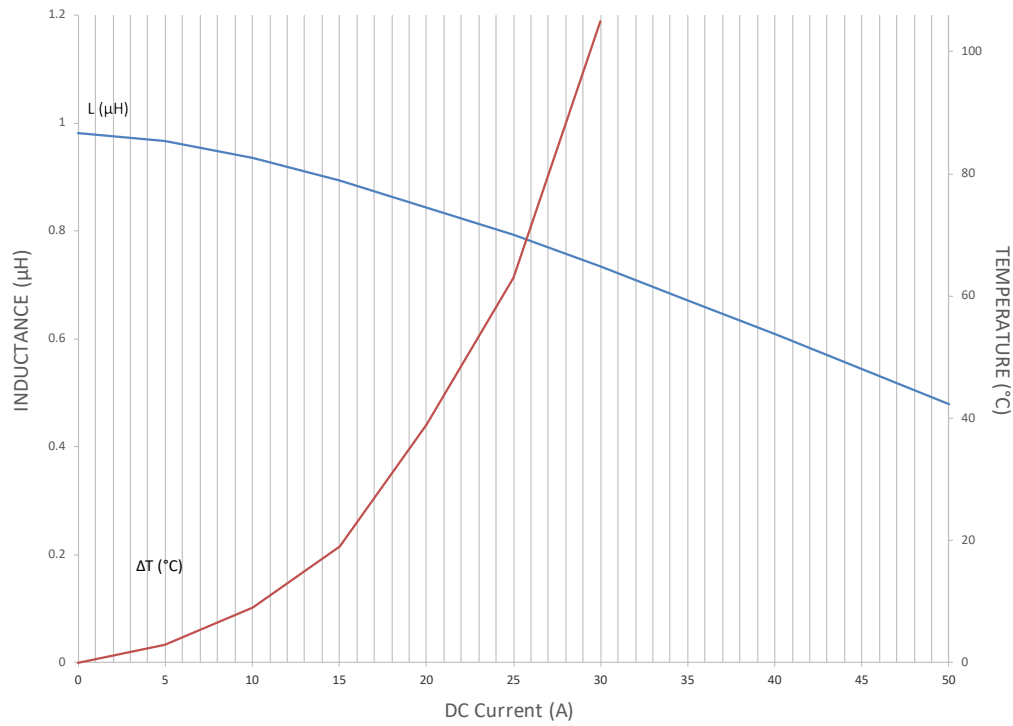
I&T Curve
