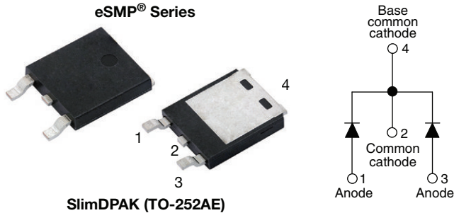
SlimDPAK (TO-252AE)
