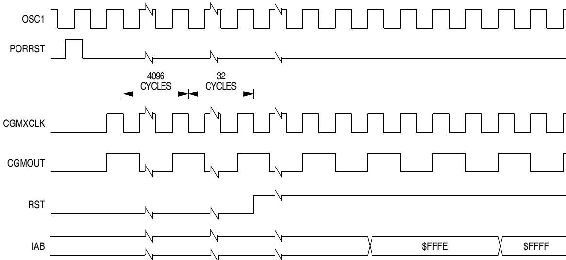
Figure 14-6. POR Recovery
