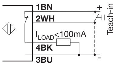
Fig. 6 PNP NC
