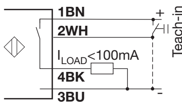
Fig. 4 PNP NO
