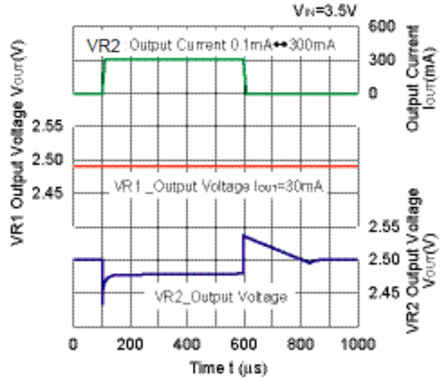
2.5V(VR2)
