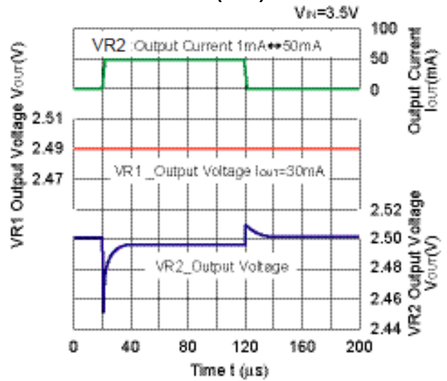
2.5V(VR2)
