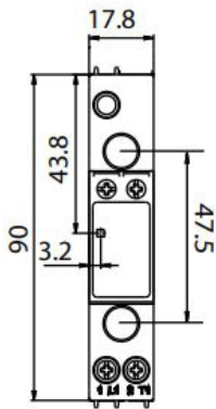
RGS...KGU
