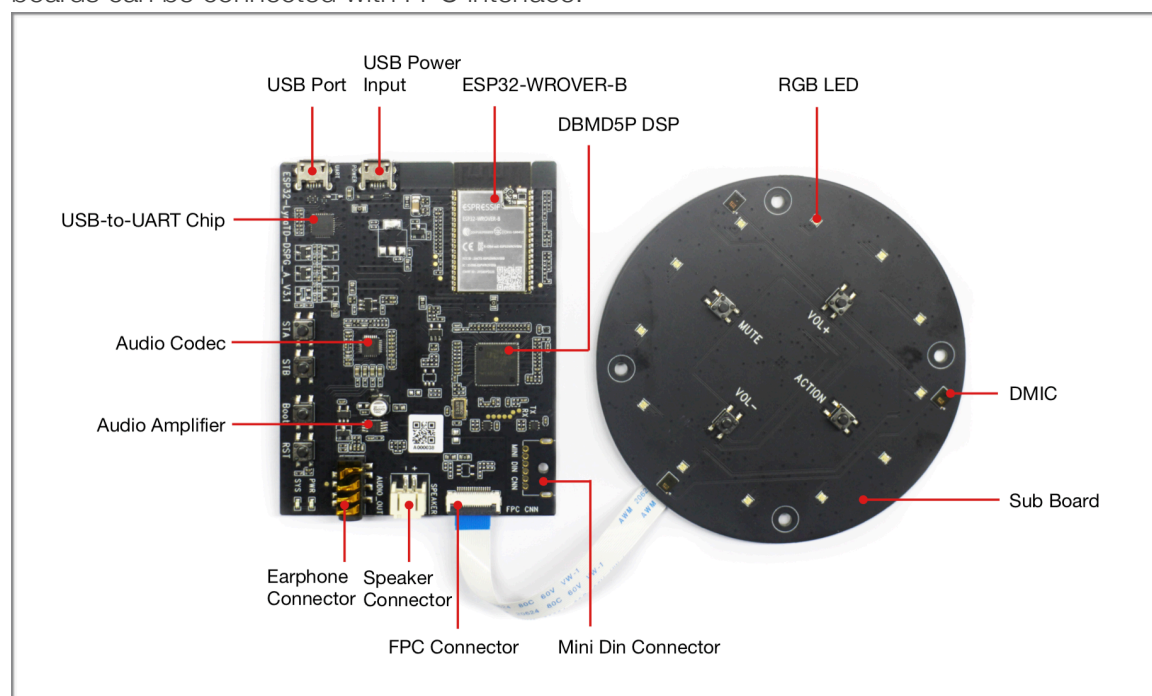
Figure 1-1. ESP32-LyraTD-DSPG Layout
