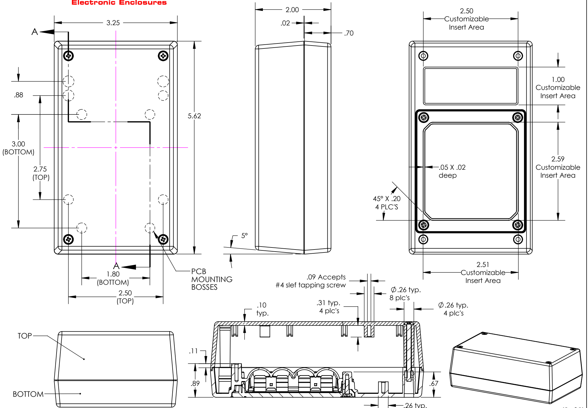
SECTION A-A
