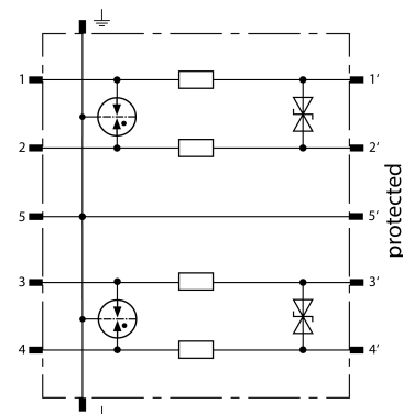
Prinzipschaltbild
