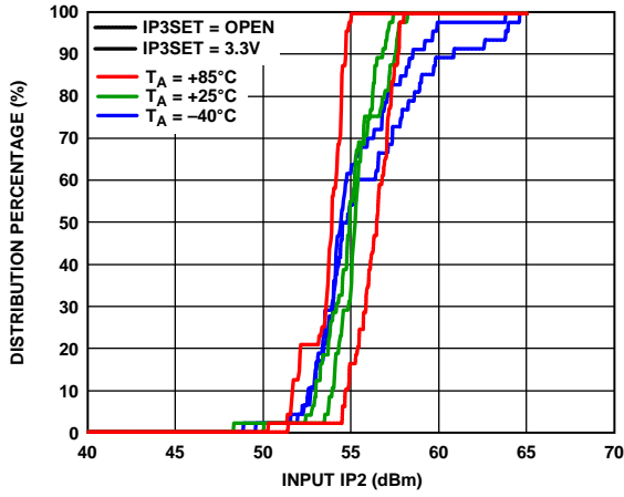
Figure 27. Input IP2
