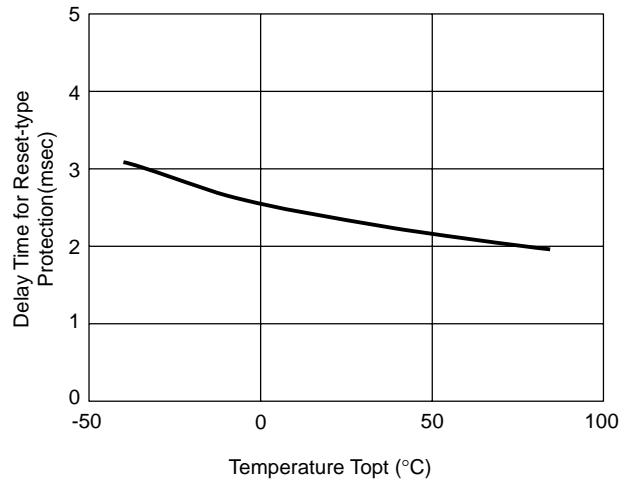
R1223N332H V_{IN}=4.5V
