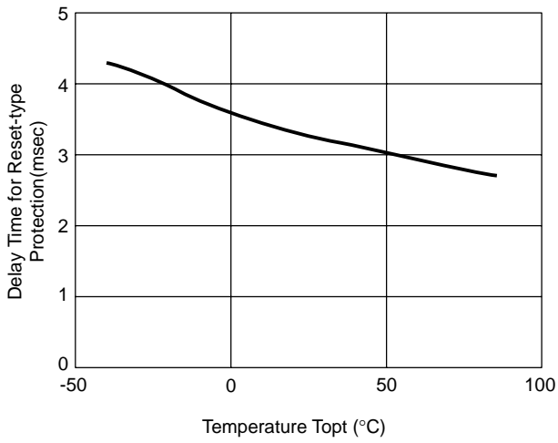
R1223N332G V_{IN}=4.5V
